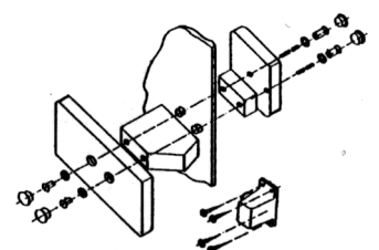
Explosionszeichnung Türgriff bei Ganzglastür
