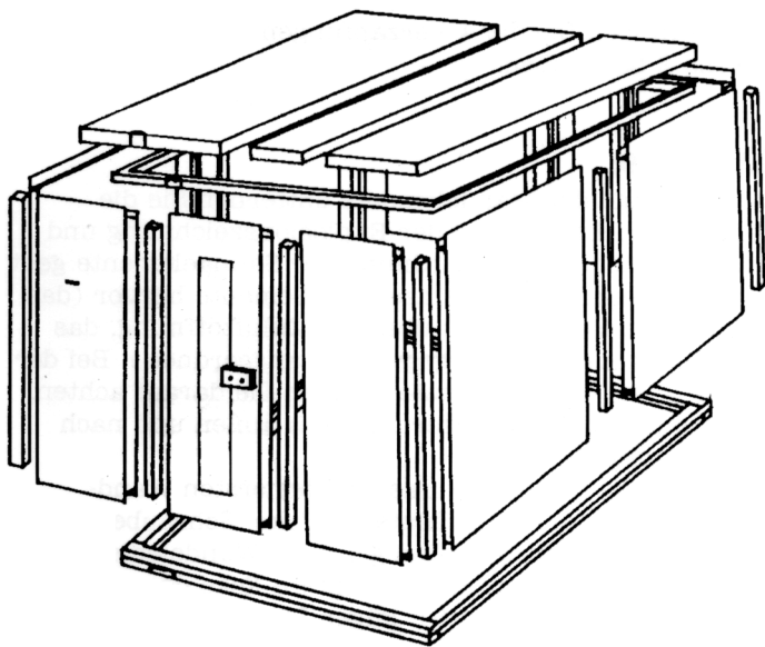
Explosionszeichnung für größere Anlagen mit zusätzlichem Dachelement
