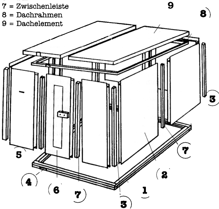
Explosionszeichnung
