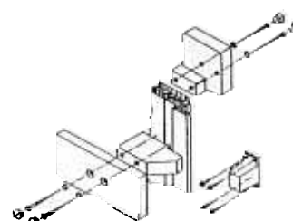
Explosionszeichnung Türgriff
